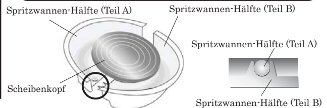
Spritzwannen-Hälfte (Teil B)
